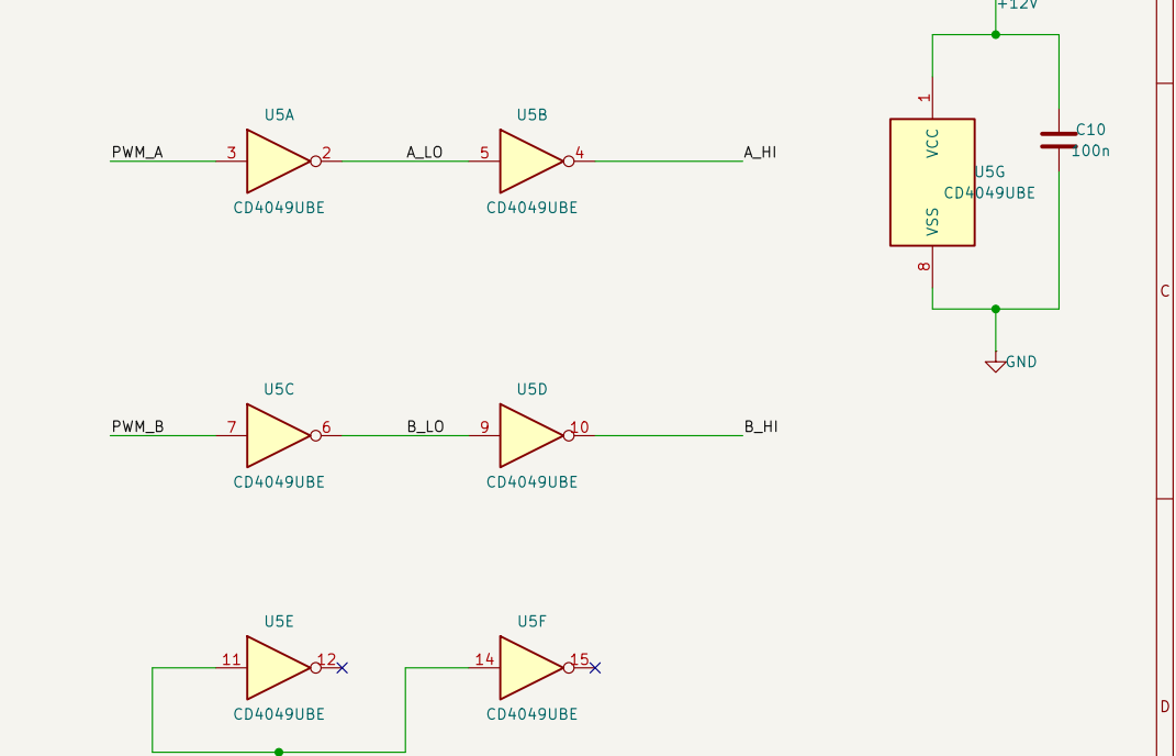
E1 Complement generation (CD4049)
